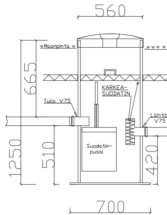
Suodatinkaivo
