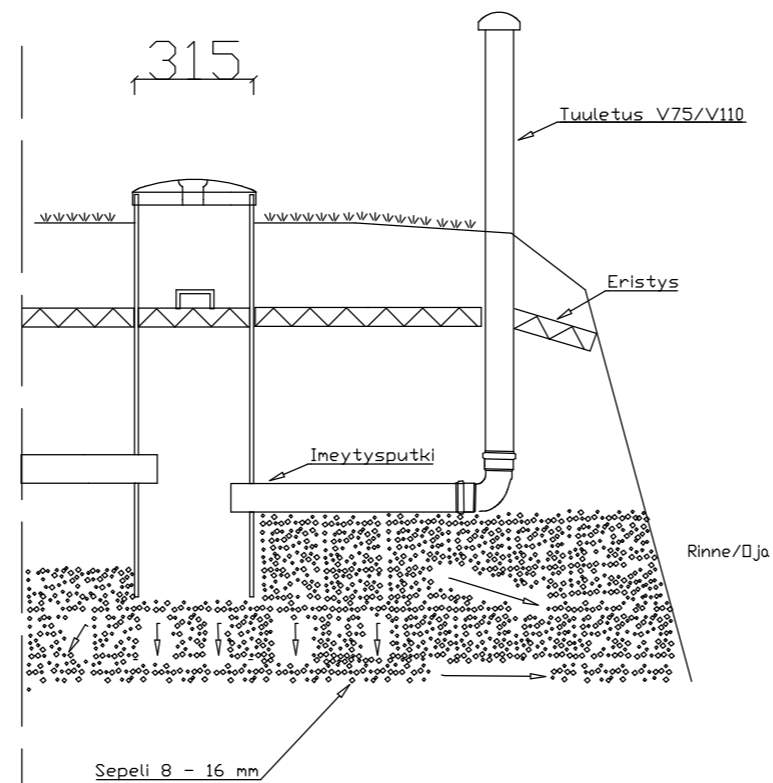
Imeytyskaivo
