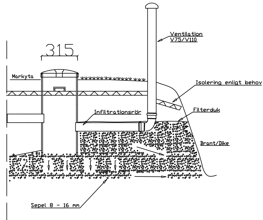
Infiltrationsbrunn
