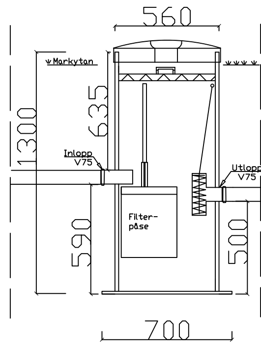
Filtreringsbrunn
